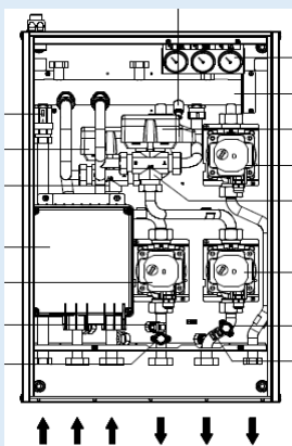
SKEMA e aparatit DIM A/2BT ErP 1 + 2 ZONA
